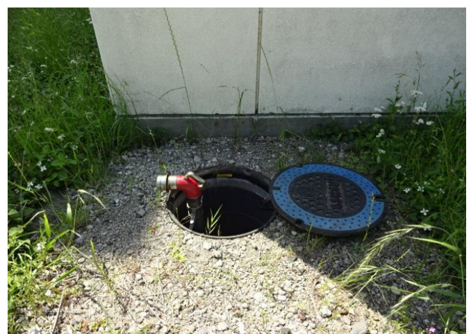
給水栓(φ500mm蓋)
