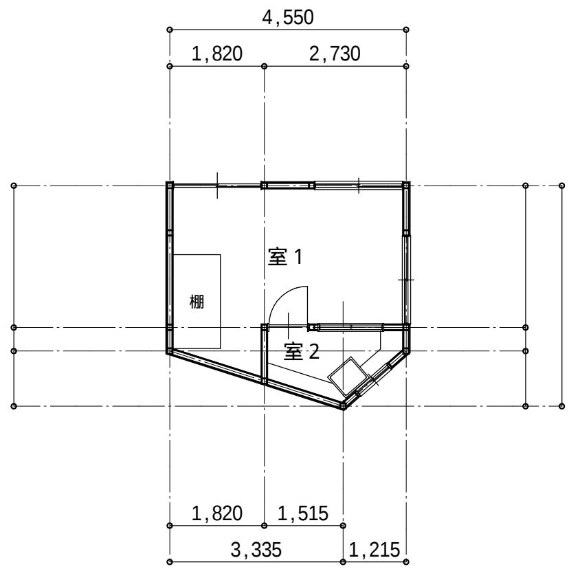
住宅付属棟 平面図
