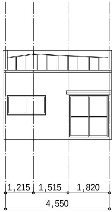
住宅付属棟 南一立面図
