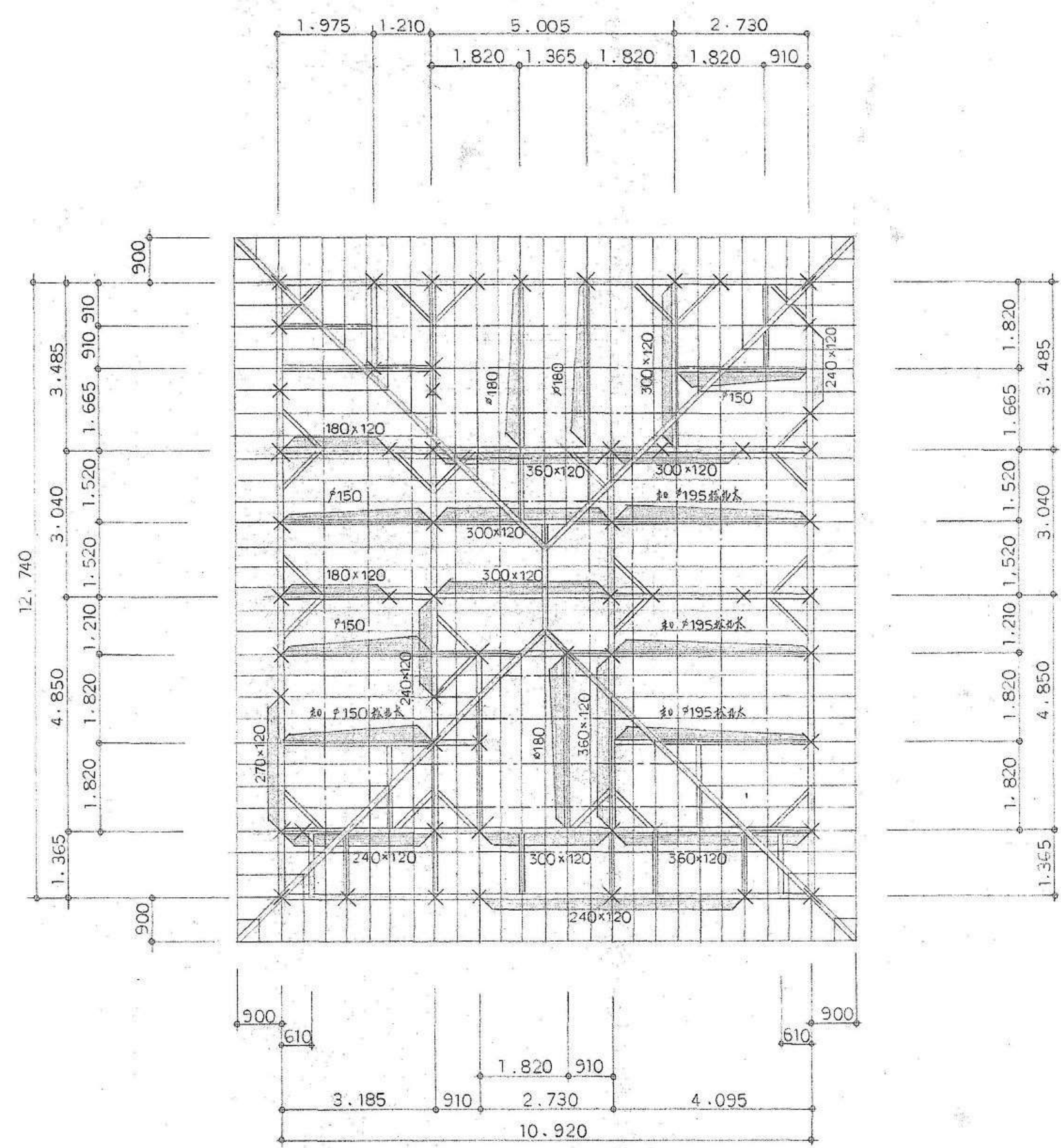
2階小屋伏図 1:100
