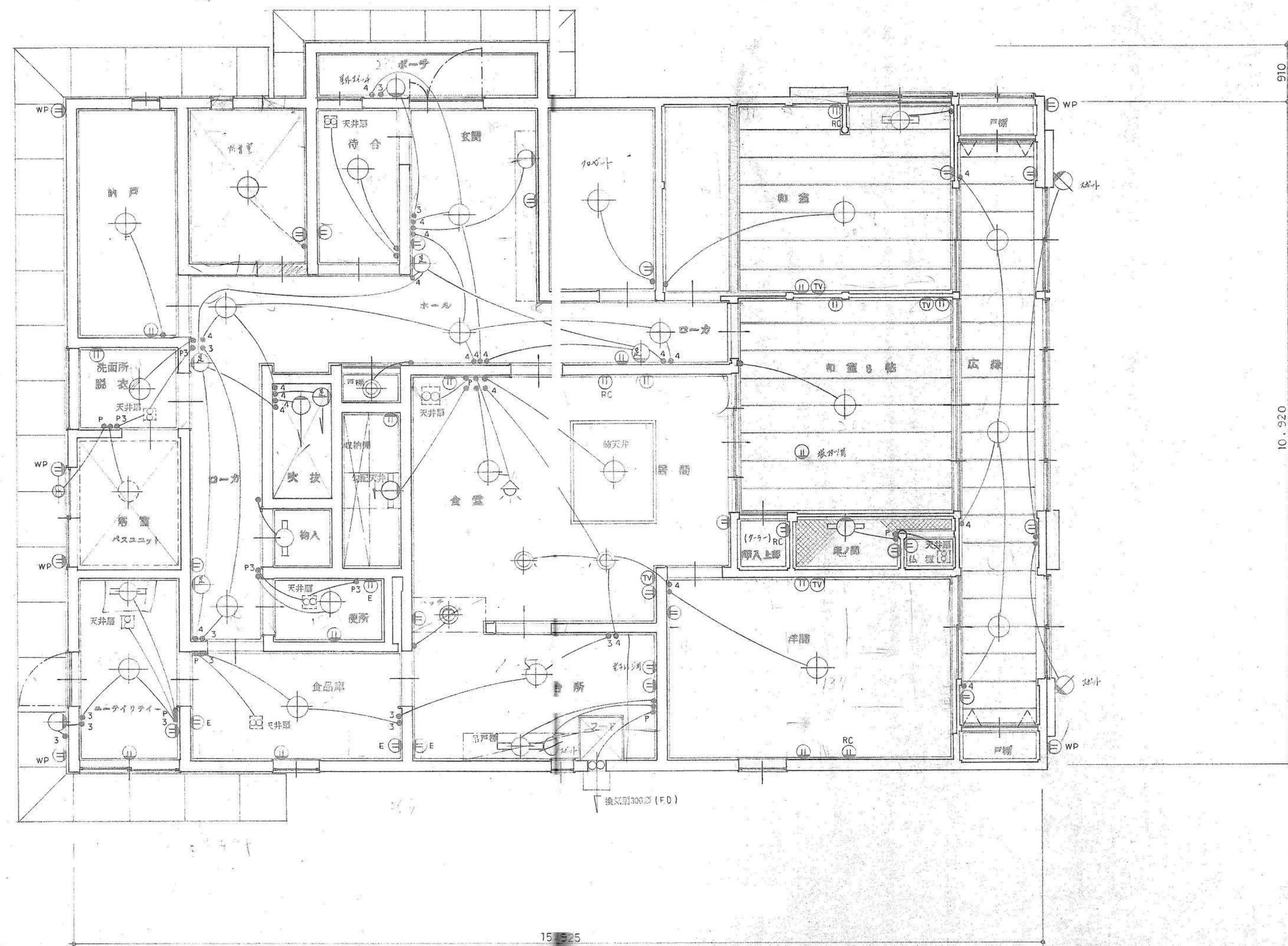
1階天井伏図・照明配置図 1/50
