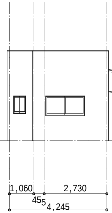
住宅付属棟 西一立面図
