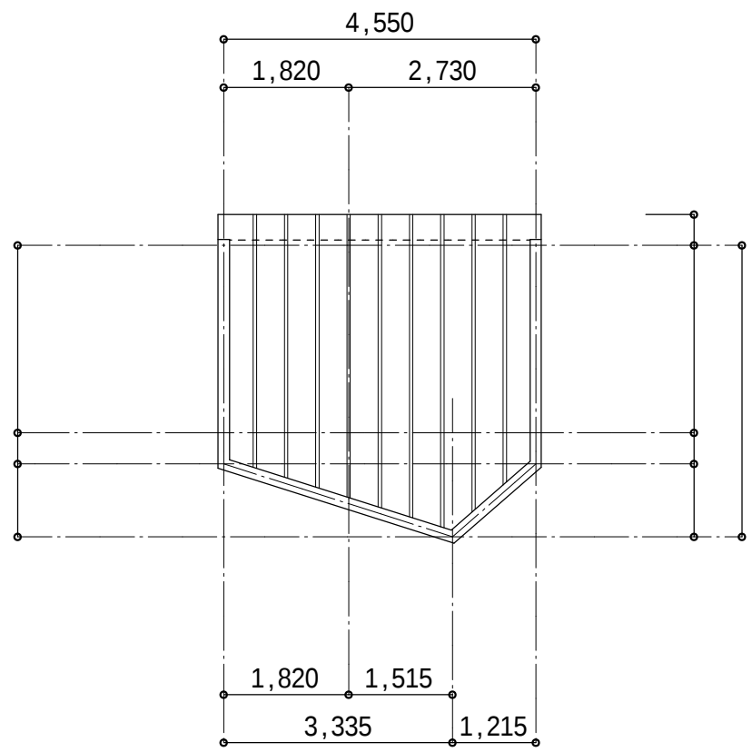
住宅付属棟 屋根伏図
