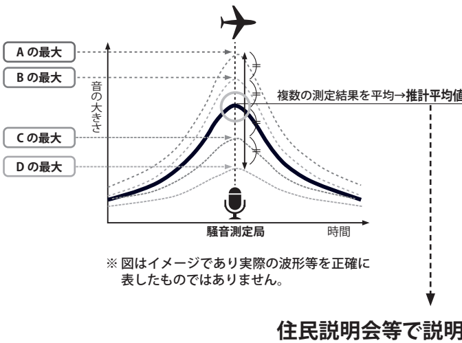
着陸時(経路直下)の騒音レベル(L_Amax[dB(デシベル)])
