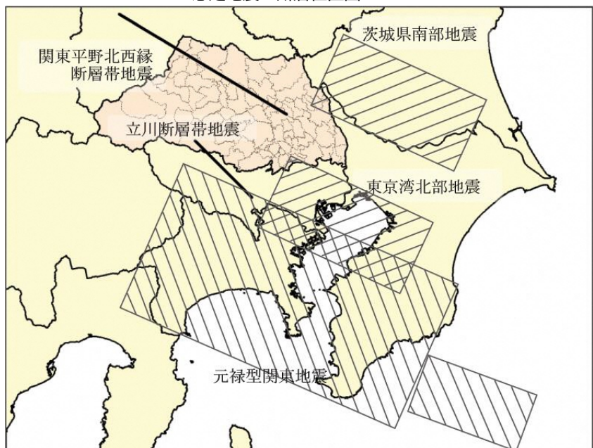
想定地震の断層位置図
